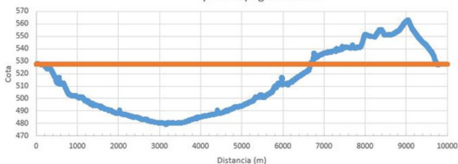
perfil topográfico 10Km
